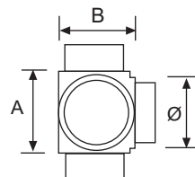
EMPALME EN "X" DE 90° 90° "X" TUBE CONNECTOR RACCORD EN CROIX, 90°
