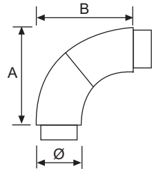
UNIÓN/DESVÍO VARIABLE ADJUSTABLE ELBOW RACCORD DE JONCTION VARIABLE
