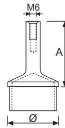
APOYO DE ATORNILLAR RECTO SIMPLE WELDING TUBE SUPPORT SUPPORT POUR VISSER
