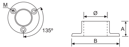
BASE ESFÉRICA ROUND BASE PLATE EMBASE MURALE SPHÉRIQUE
