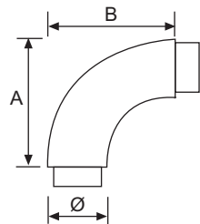
EMPALME REDONDO DE 90° RADIUSED ELBOW RACCORD 90° ROND
