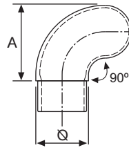
TERMINAL CURVADO ROUNDED HANDRAIL 90° ENDING EMBOUT À COLLER COURBÉ
