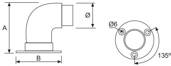
CODO DE 90° CON SOPORTE 90° ELBOW WITH BASE SUPPORT MUR COUDE 90°
