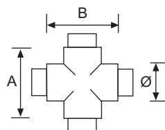
EMPALME EN "X" "X" TUBE CONNECTOR RACCORD EN CROIX
